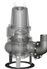
Curva flangiata con portagomma N4 Base di sostegno P8 Flanged hose connection N4 Foot support P8
